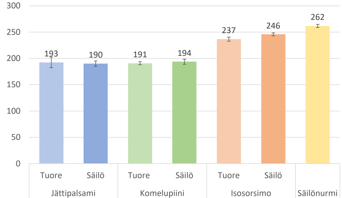
Metaanituotto kuiva-ainetta kohden [m 3 /t]
